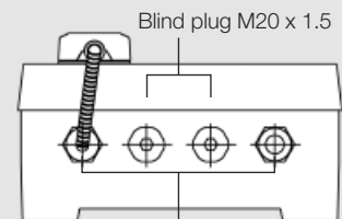
Blind plug M20 x 1.5 Cable gland M20 x 1.5
